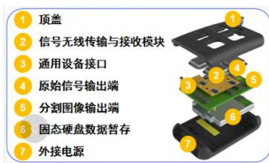
图 2-3：产品结构图
