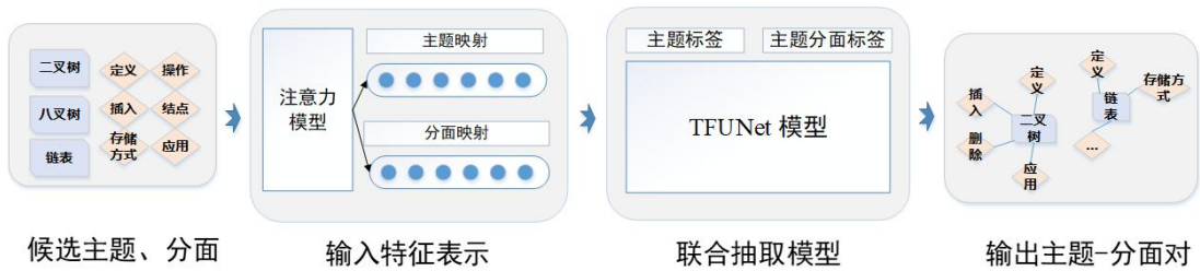
图 2-14：知识图谱主题分面树生成办法
