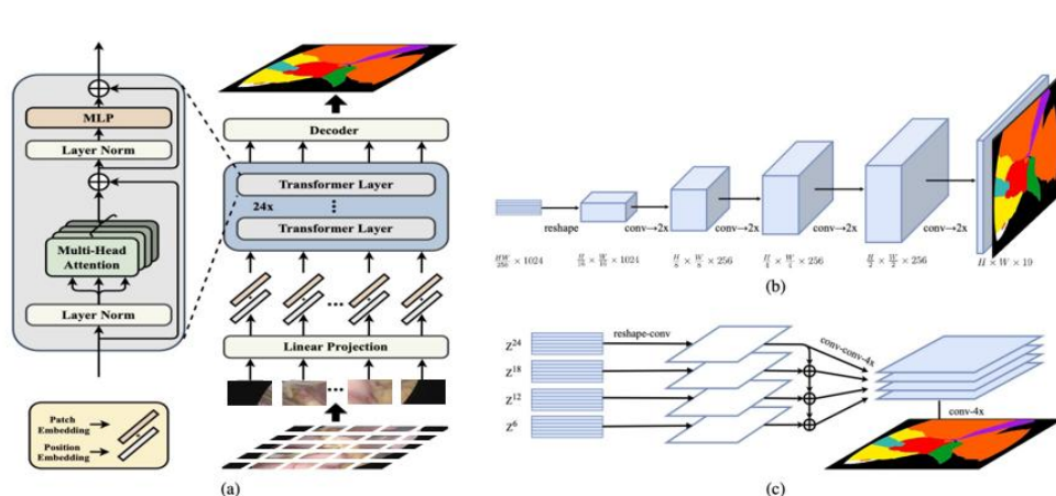
图 2-11: 改进 Yun-Transformer 算法流程图
