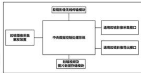
图 25 术腹腔镜图像采集装置结构示意图
